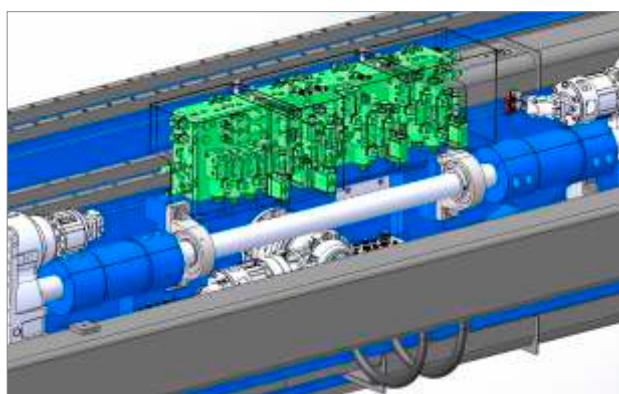
Gruppo valvole proporzionali Group of proportional valves
