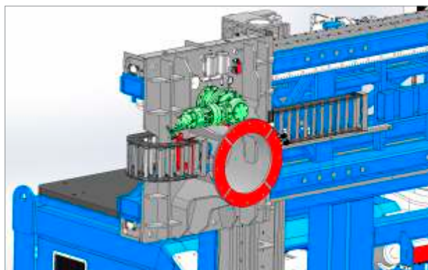
Motoriduttore traslazione carro portatesta - asse X2 Head carrying trolley travel gearbox - X2 axis
