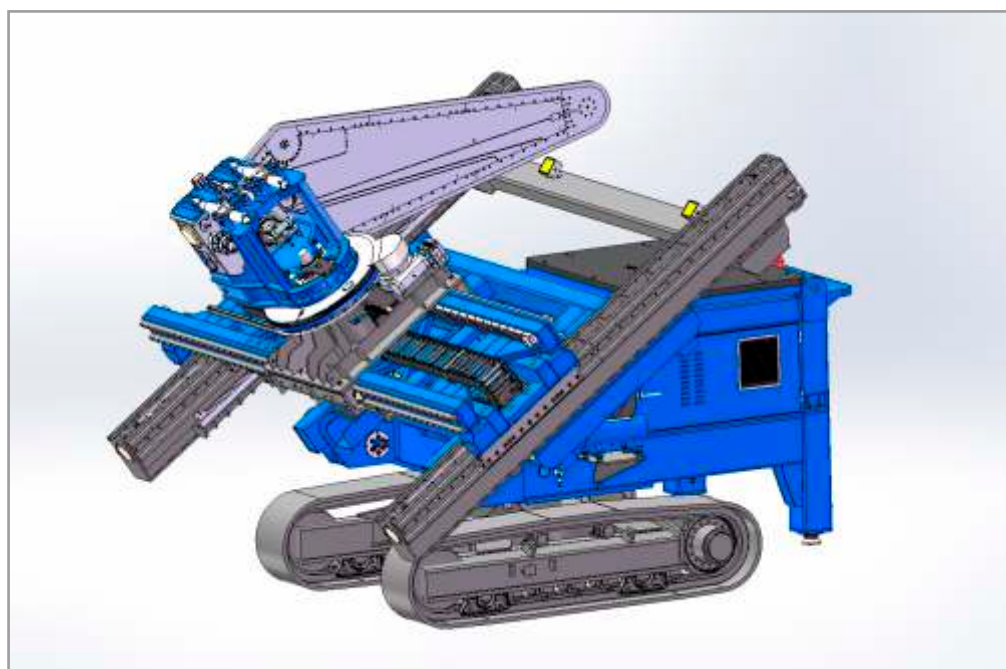
Macchina configurata per lo spostamento. / Machine configured for the movement.
