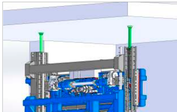
Stabilizzatori superiori sulle colonne del telaio portante Upper positioning hydraulic jacks on two columns of the portal
