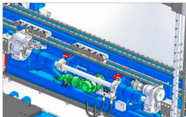
Motorizzazione - asse X1 Driving unit - X1 axis
