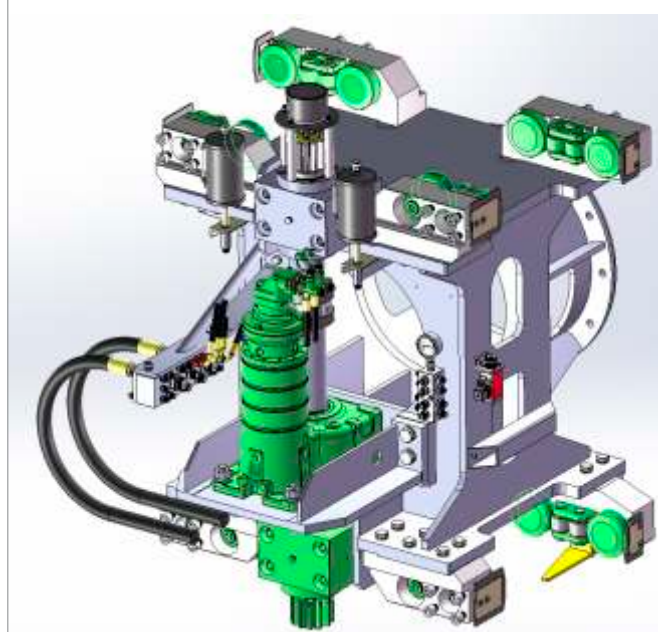
La testa operatrice è montata su un carrello che scorre su una trave orizzontale per mezzo di otto ruote di guida e otto pattini di contrasto. La trasmissione è realizzata con sistema pignone - cremagliera.
