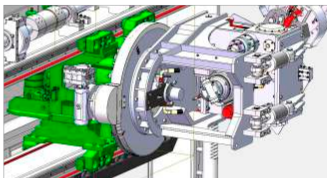
Trasmissione carro testa Head trolley transmission
