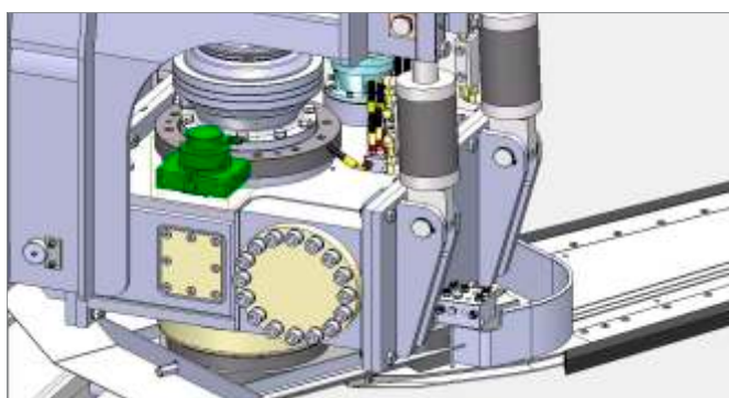
Encoder rotazione lama Arm rotation encoder
