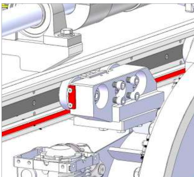
Dettaglio guide Hoesch per traslazione orizzontale con riporto in hardox. Detail of the Hoesch guides for horizontal translation with hardox cover.
